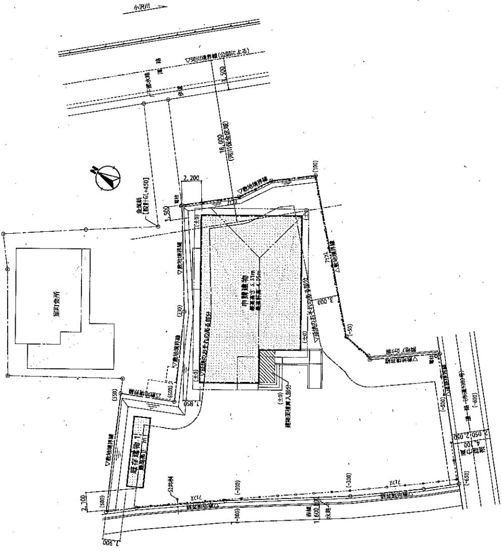
配置図 S=1/200
