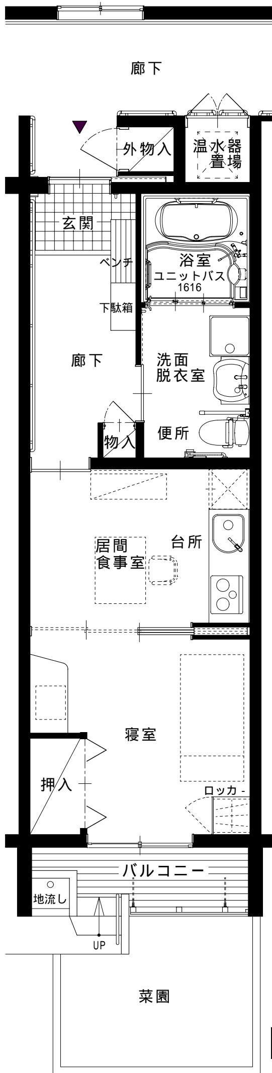
1人用住戸間取平面図
