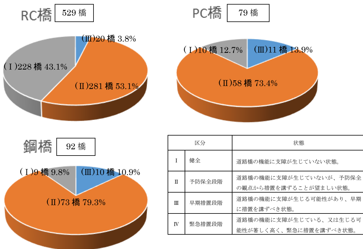
図 5 橋(上部工)の部分の構造材料種別の点検結果
