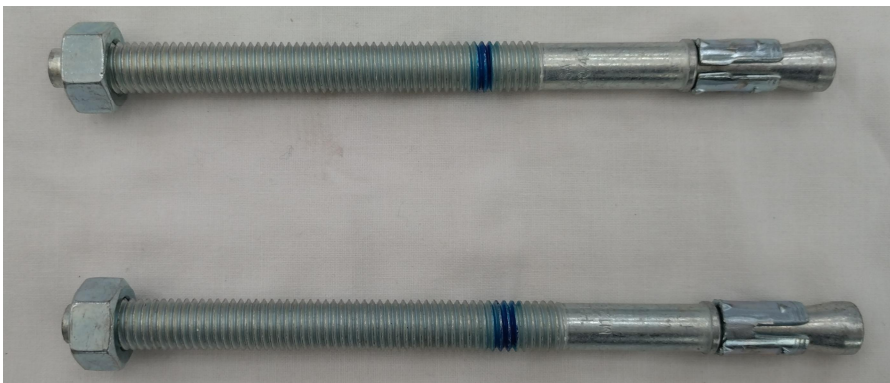
HILTI HSA M12×175 95/80/45 2本 (ワッシャーなし)
