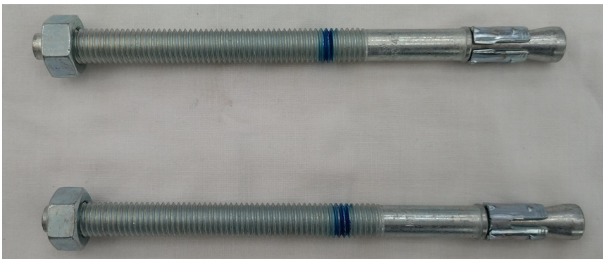
HILTI HSA M12×175 95/80/45 2本 (ワッシャーなし)
