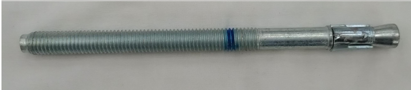
HILTI HSA M12×175 95/80/45 1本 (ワッシャー、ナットなし)
