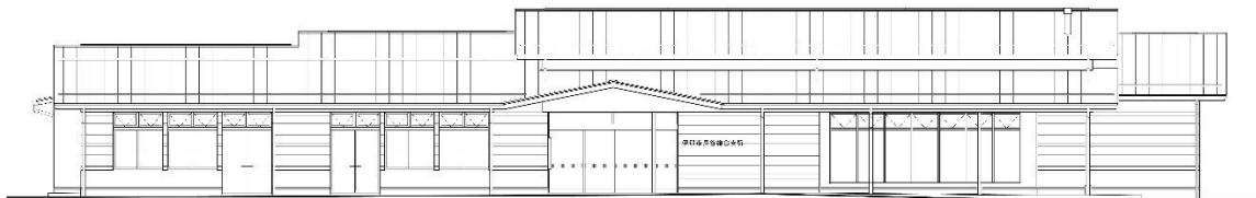
北側立面図
