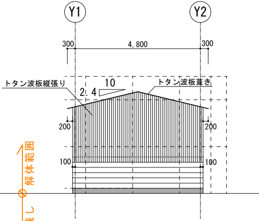
南側立面図 1/100
