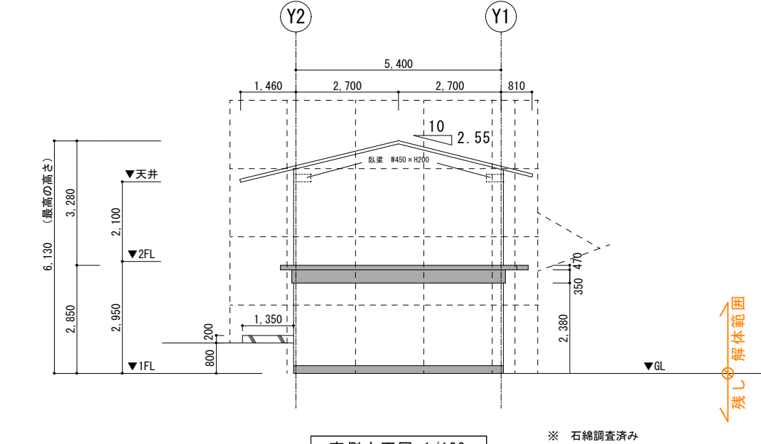
南側立面図 1/100
