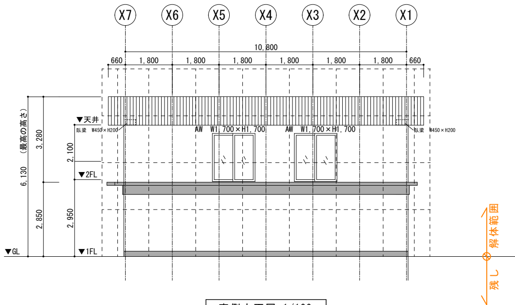
東側立面図 1/100
