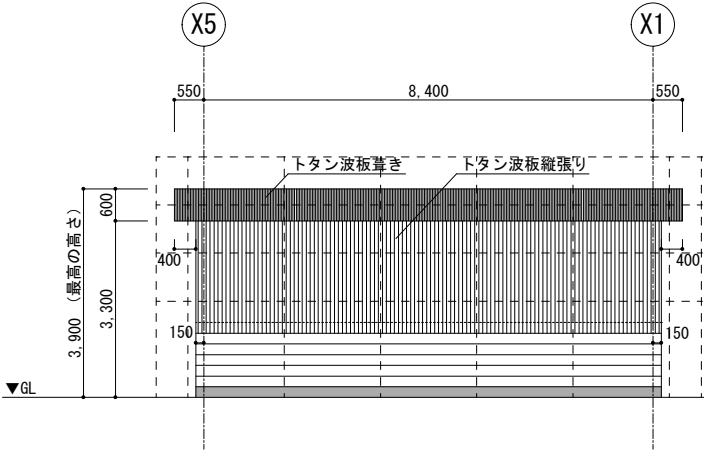
東側立面図 1/100
