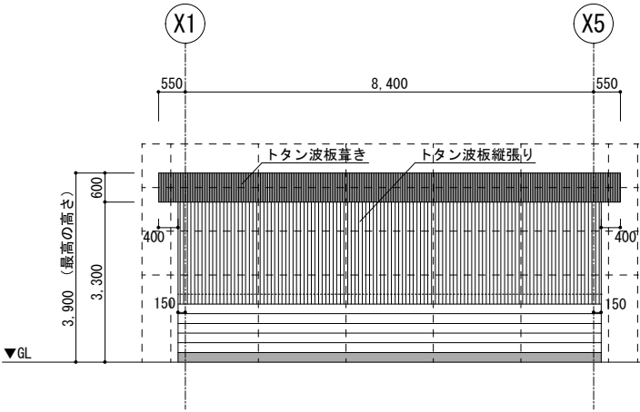
西側立面図 1/100
