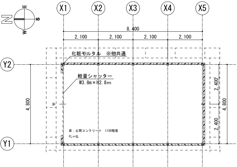
平面図 1/100
