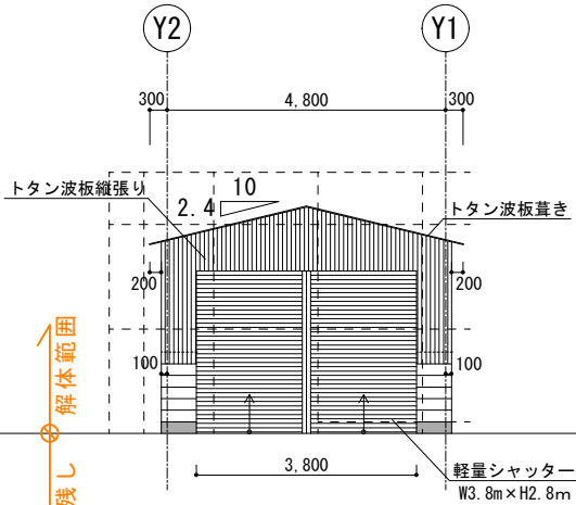
北側立面図 1/100
