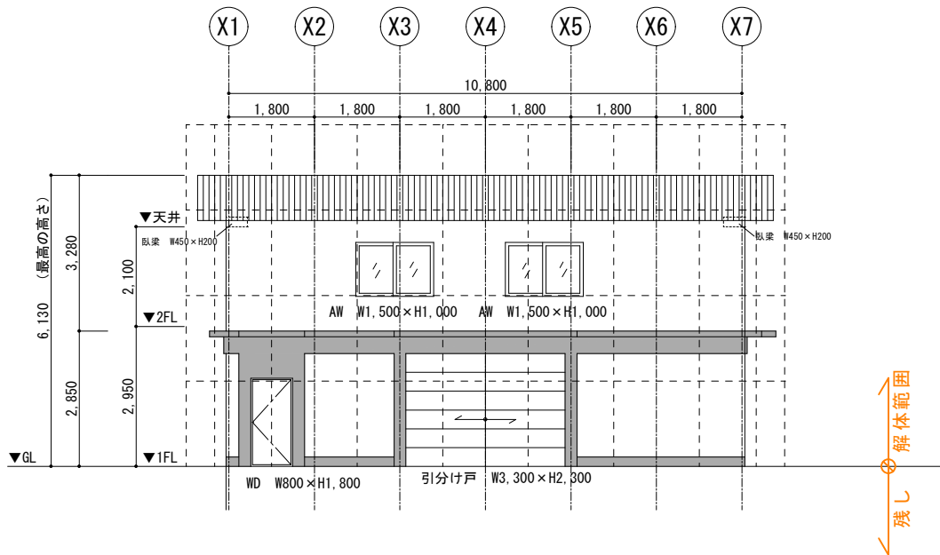
西側立面図 1/100
