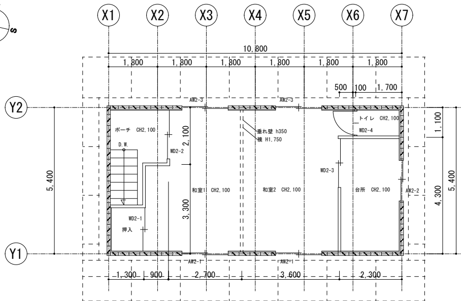
2 階平面図 1/100
