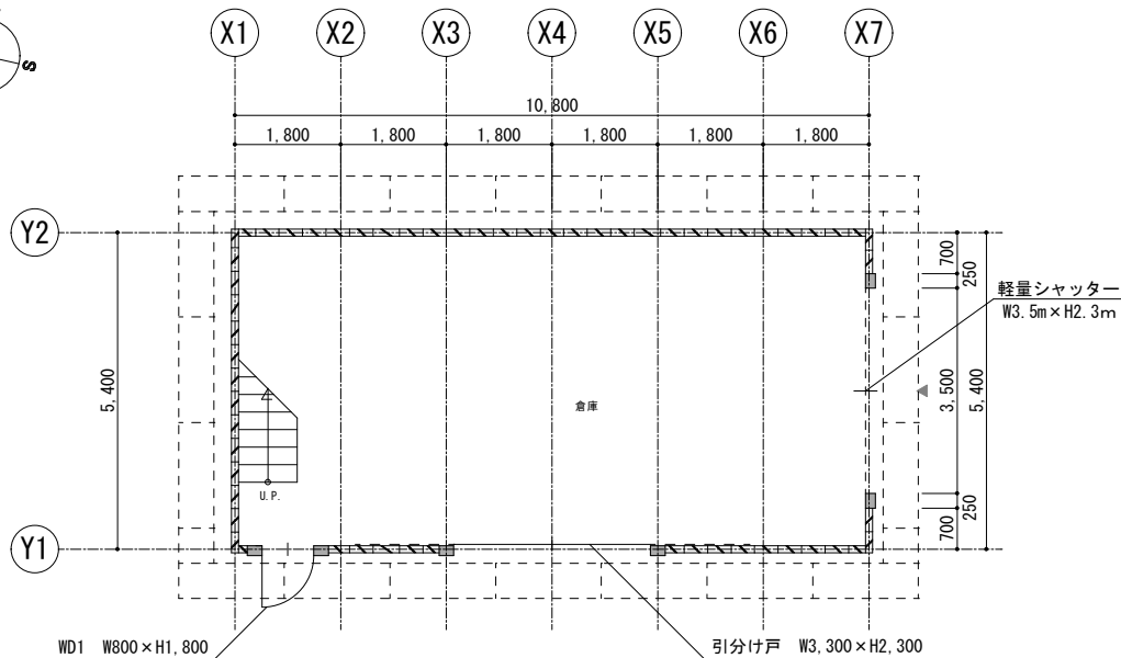
1 階平面図 1/100
