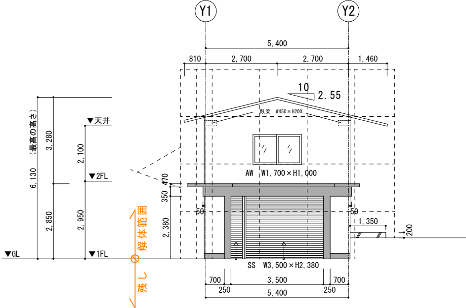
北側立面図 1/100
