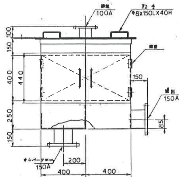
スクリーン槽詳細 S=1/10
