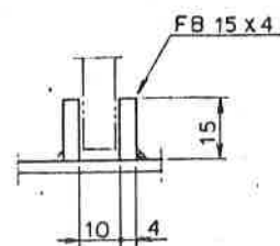
C部詳細 S=1/1
