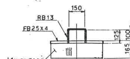
し液かご詳細 S=1/10
