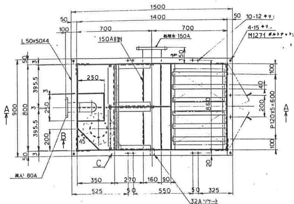
スクリーン槽詳細 S=1/10
