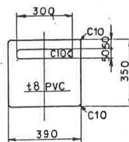
角落し詳細 S=1/10
