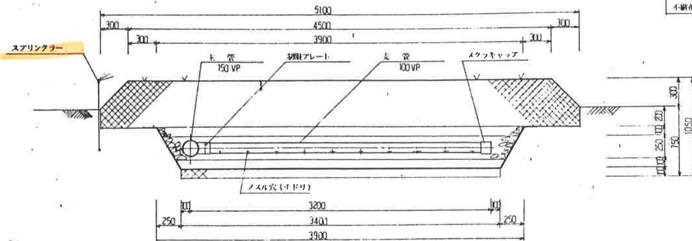
断面詳細図 S 1:20
