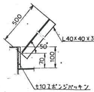
D部詳細 S=1/5
