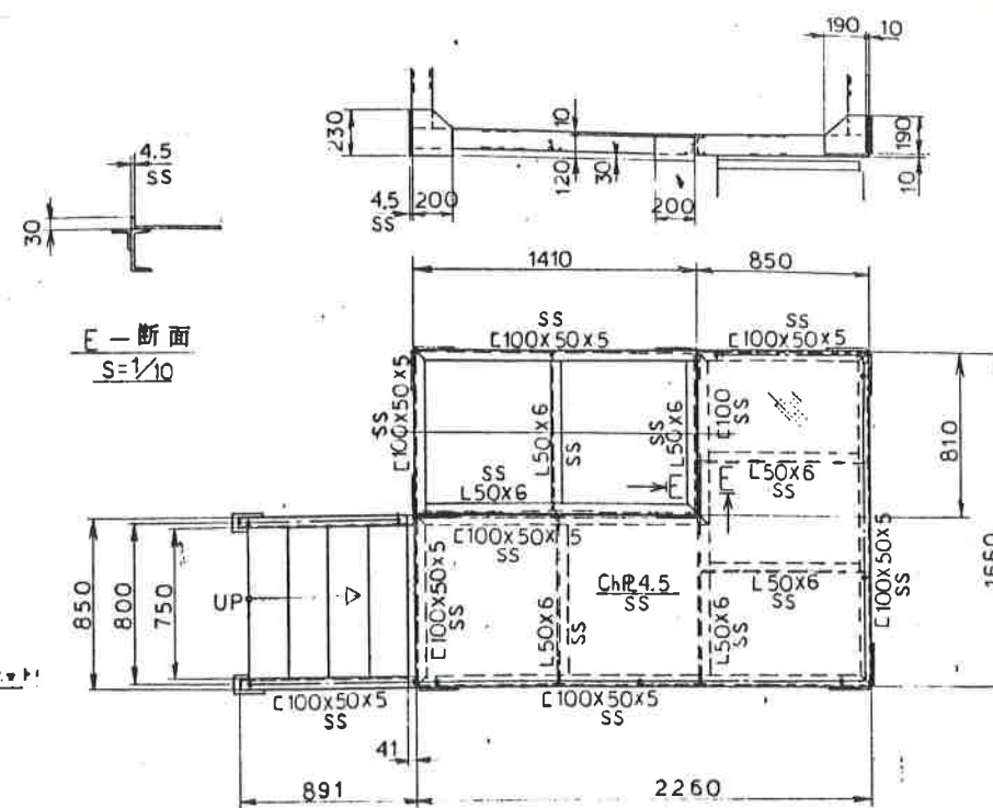
スクリーン槽架台詳細 S=1/20
