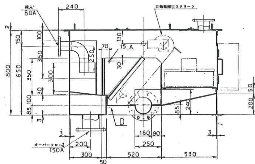
A-A断面 S=1/10
