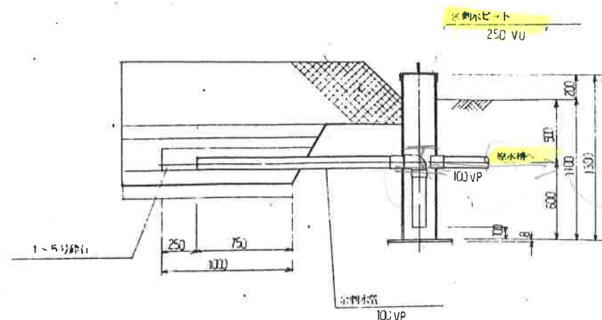
余剰水排水管部詳細図 S 1:20
