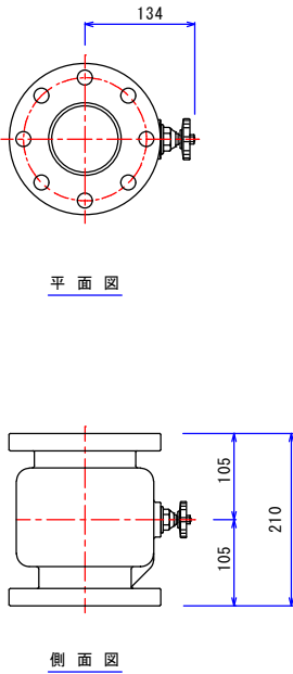
側面図
