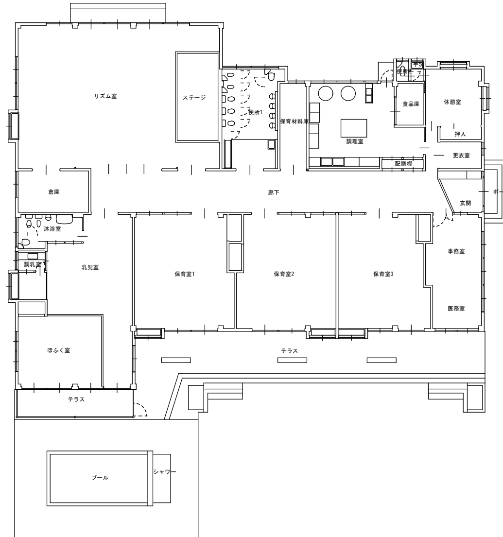
1階平面図 S=1:200
