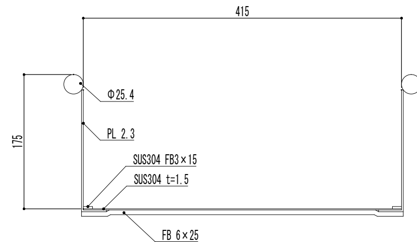
直線滑面断面図 S=1:5
