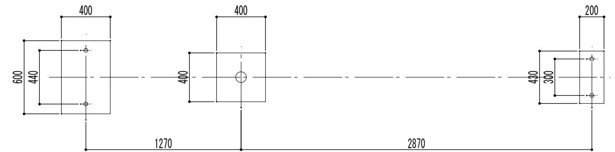
基礎伏図
