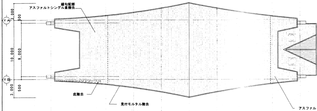
屋根伏図 (改修前) 1 / 200
