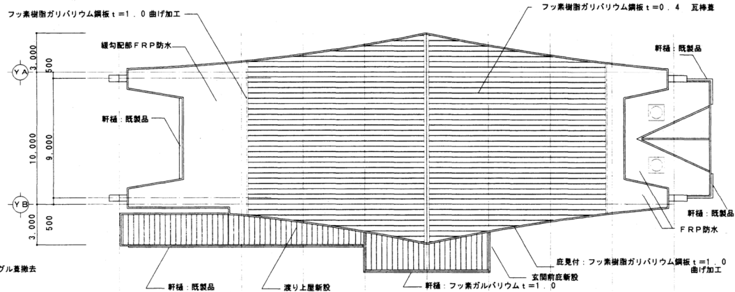
屋根伏図 (改修後) 1 / 200
