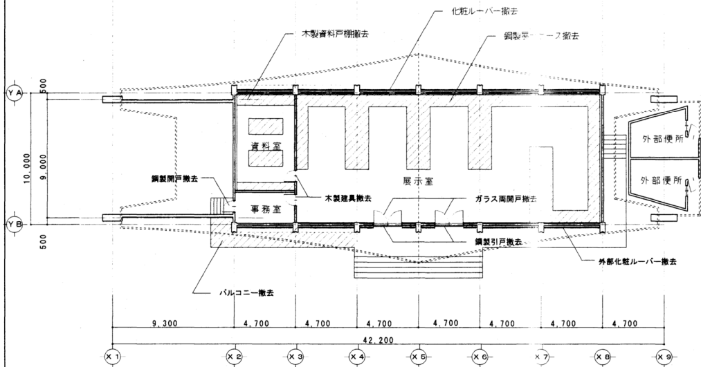
平面図 (改修前) 1 / 200
