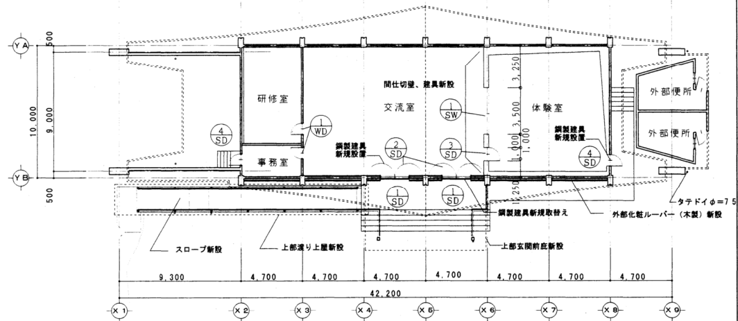
平面図 (改修後) 1 / 200
