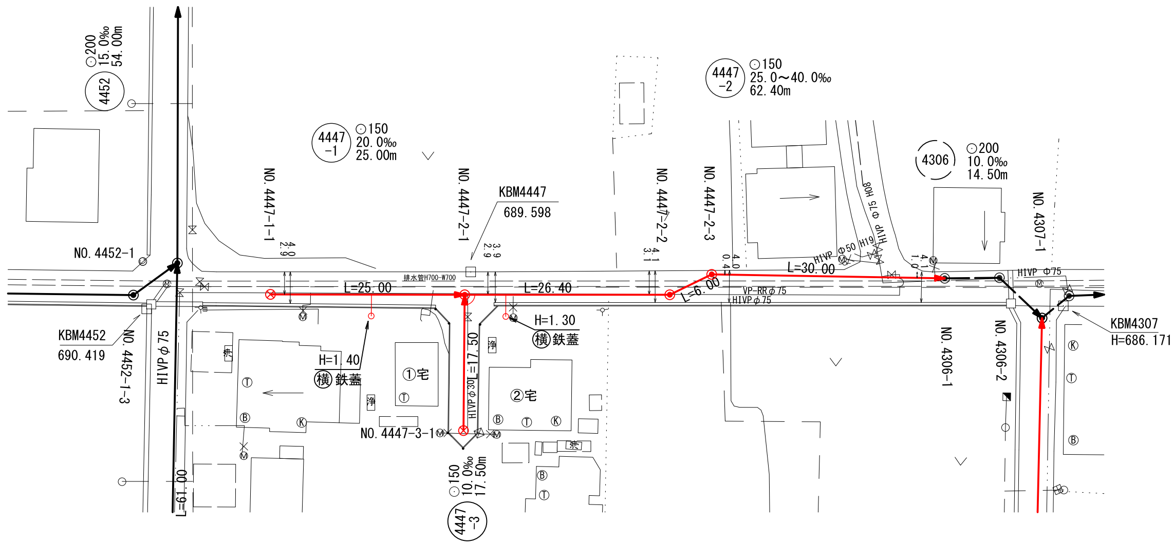
平面図 縮尺1:500
