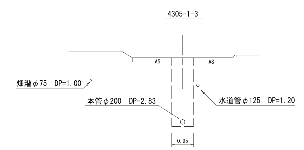
横断面図 縮尺1:100
