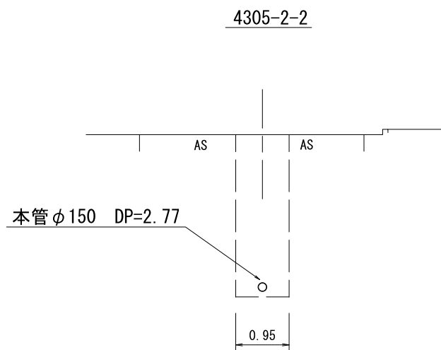
横断面図 縮尺1:100
