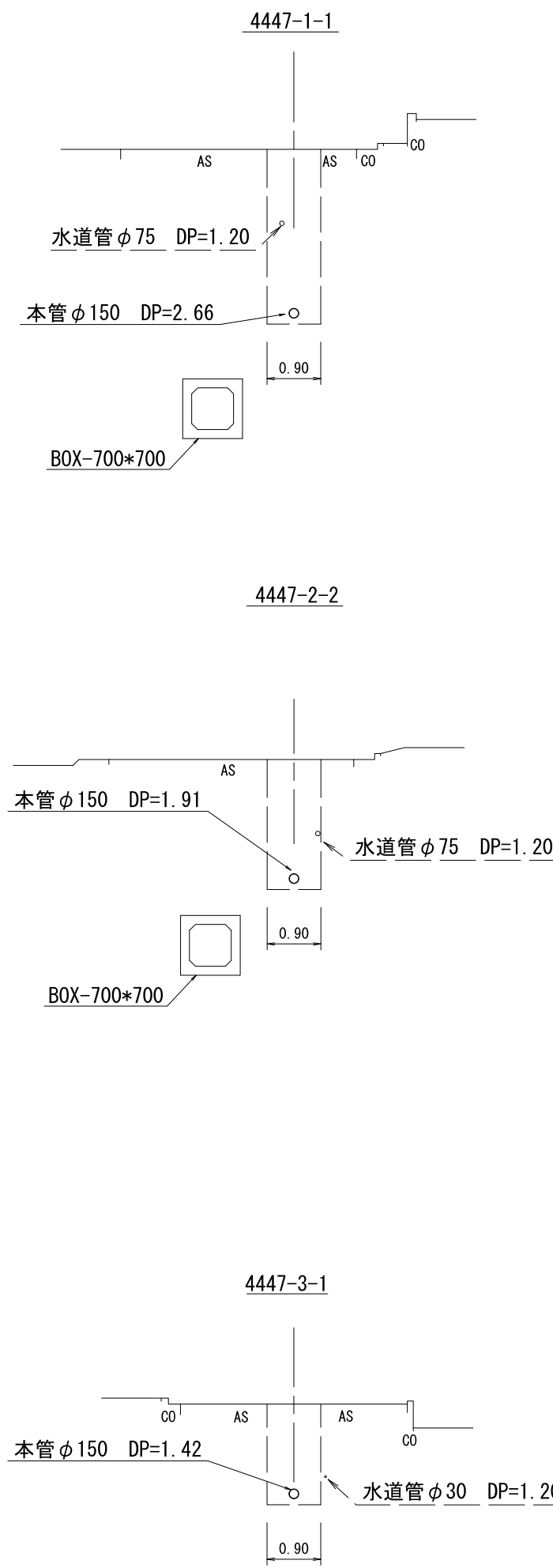
横断面図 縮尺1:100
