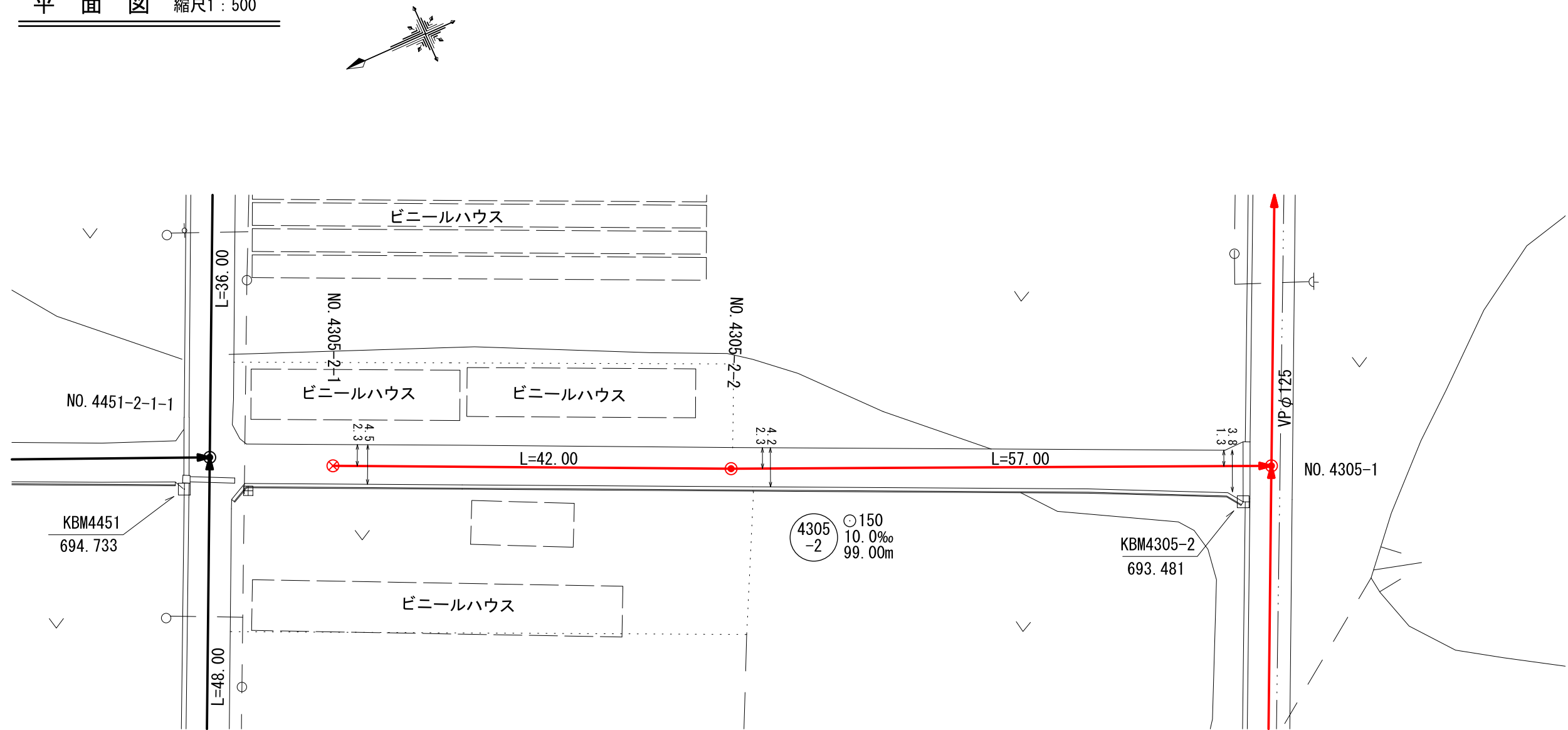
平面図 縮尺1:500
