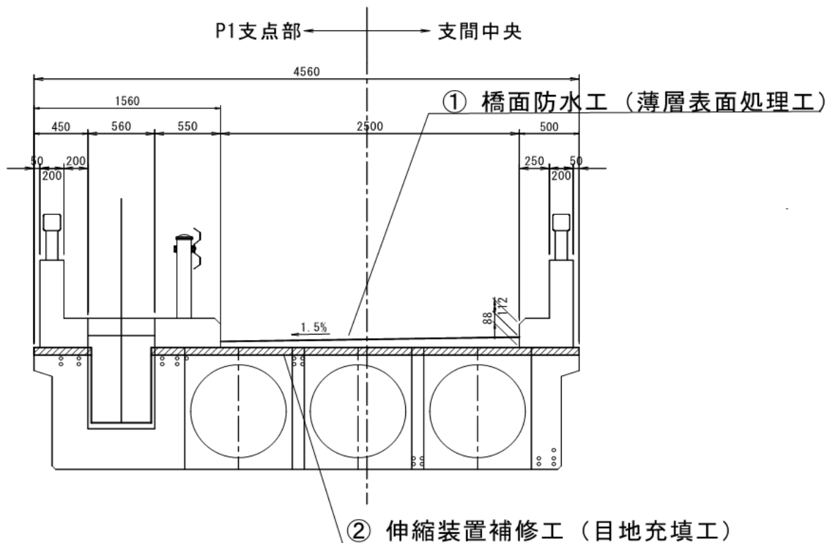
標準断面図 S=A1-1:30・A3-1:60
