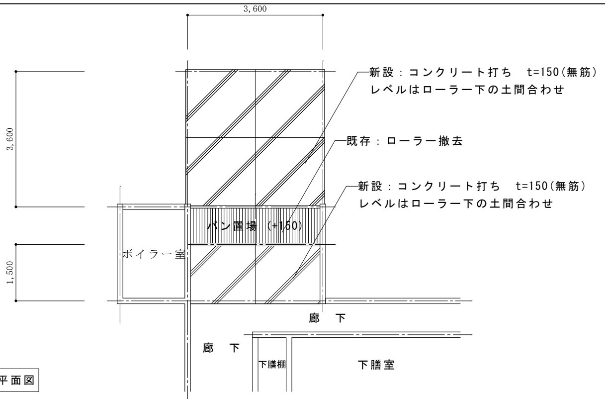
手良小学校 既存給食室 仮設配膳スペース図 1/100
