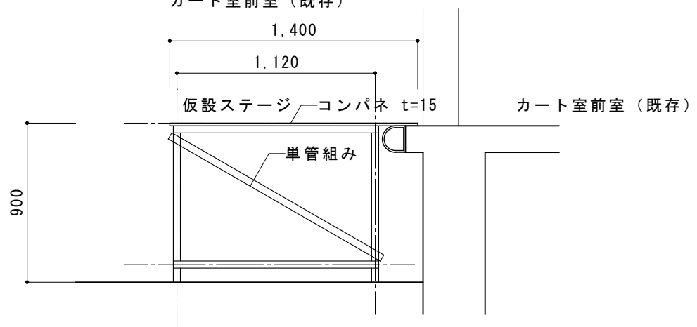
伊那中・伊那西小共同調理場 仮設ステージ図 1/30
