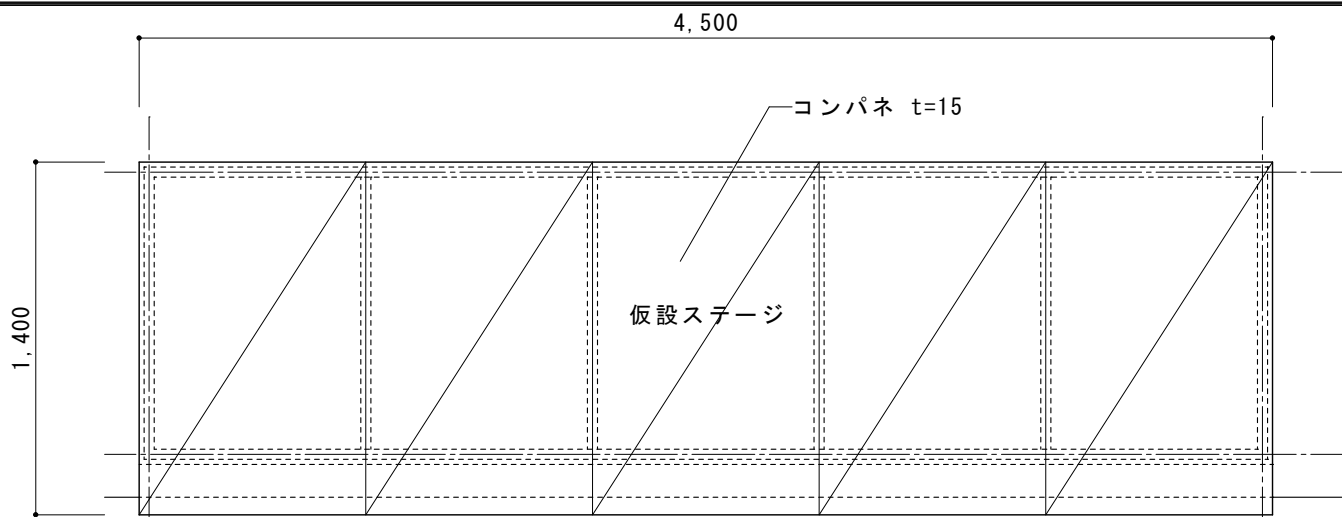
平面図
