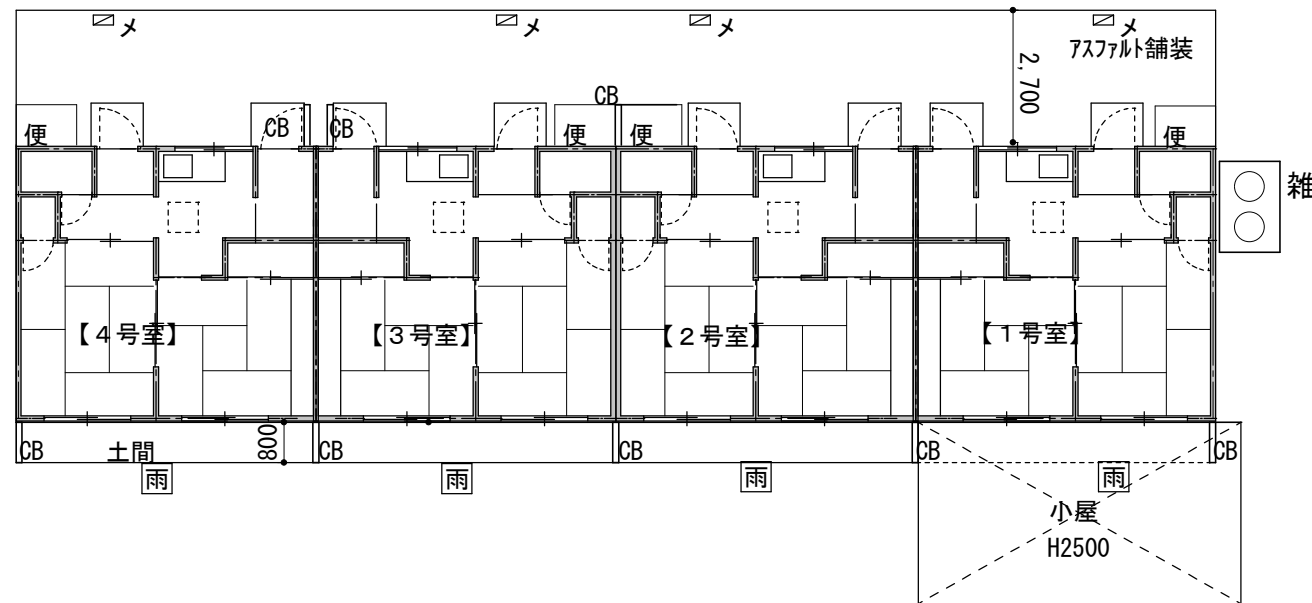
1～4号室平面図
