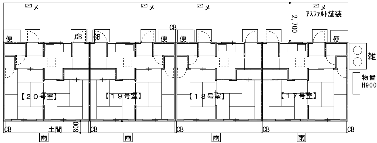
17～20号室平面図
