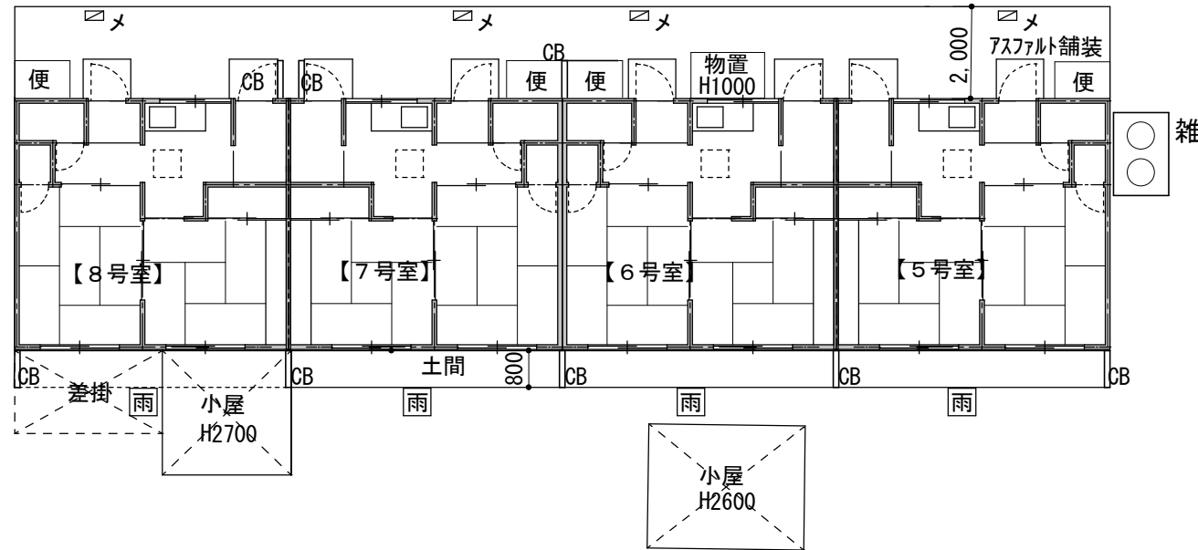
5～8号室平面図
