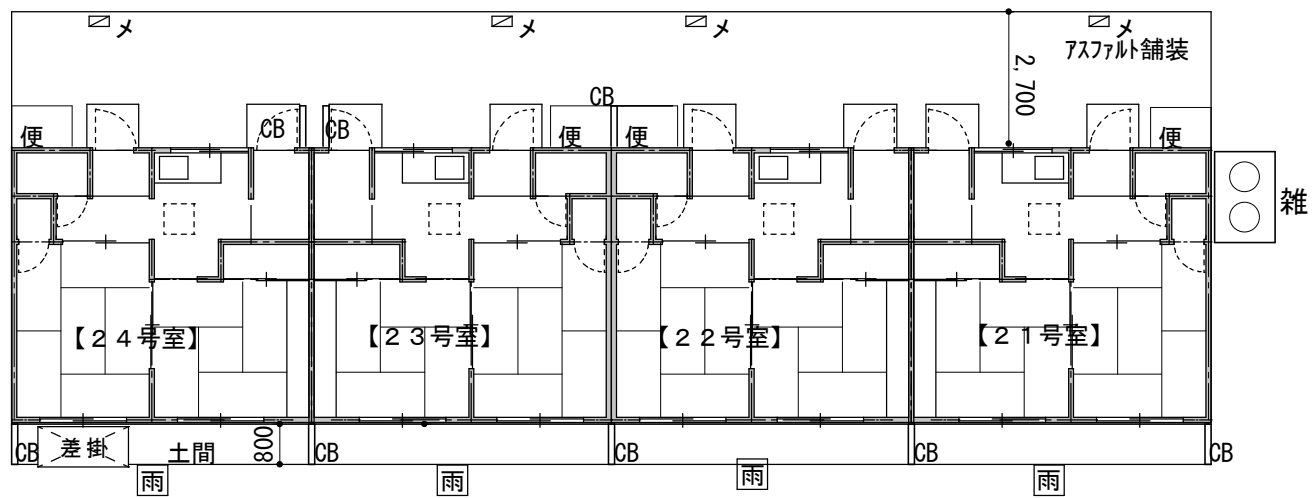
21～24号室平面図
