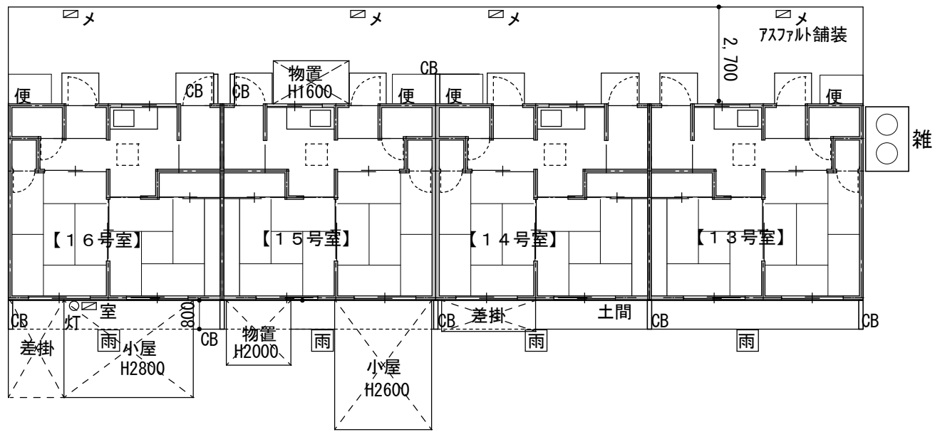
13～16号室平面図
