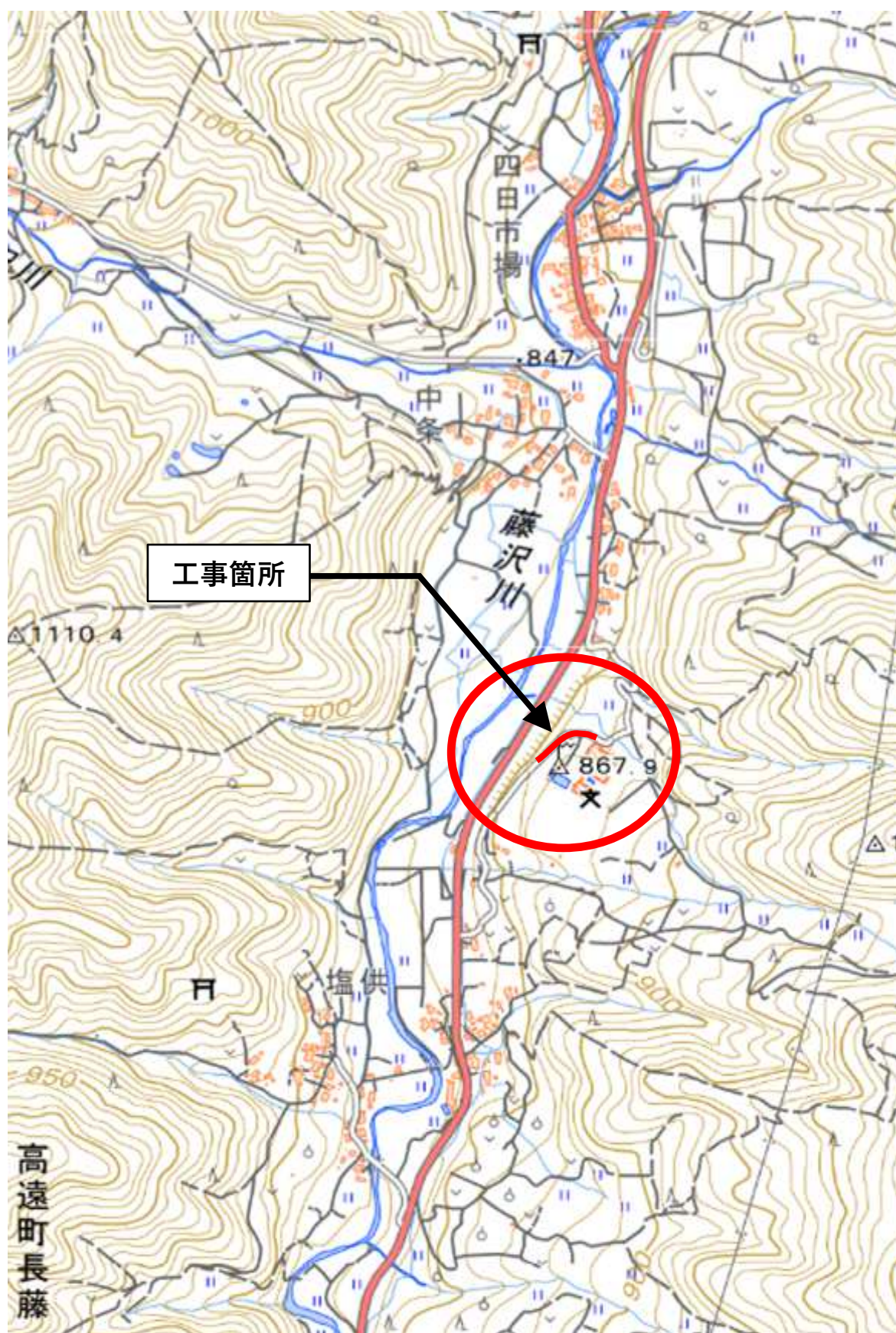
令和 8 年度 舗装修繕工事 市道宮ノ原線 施工位置図
