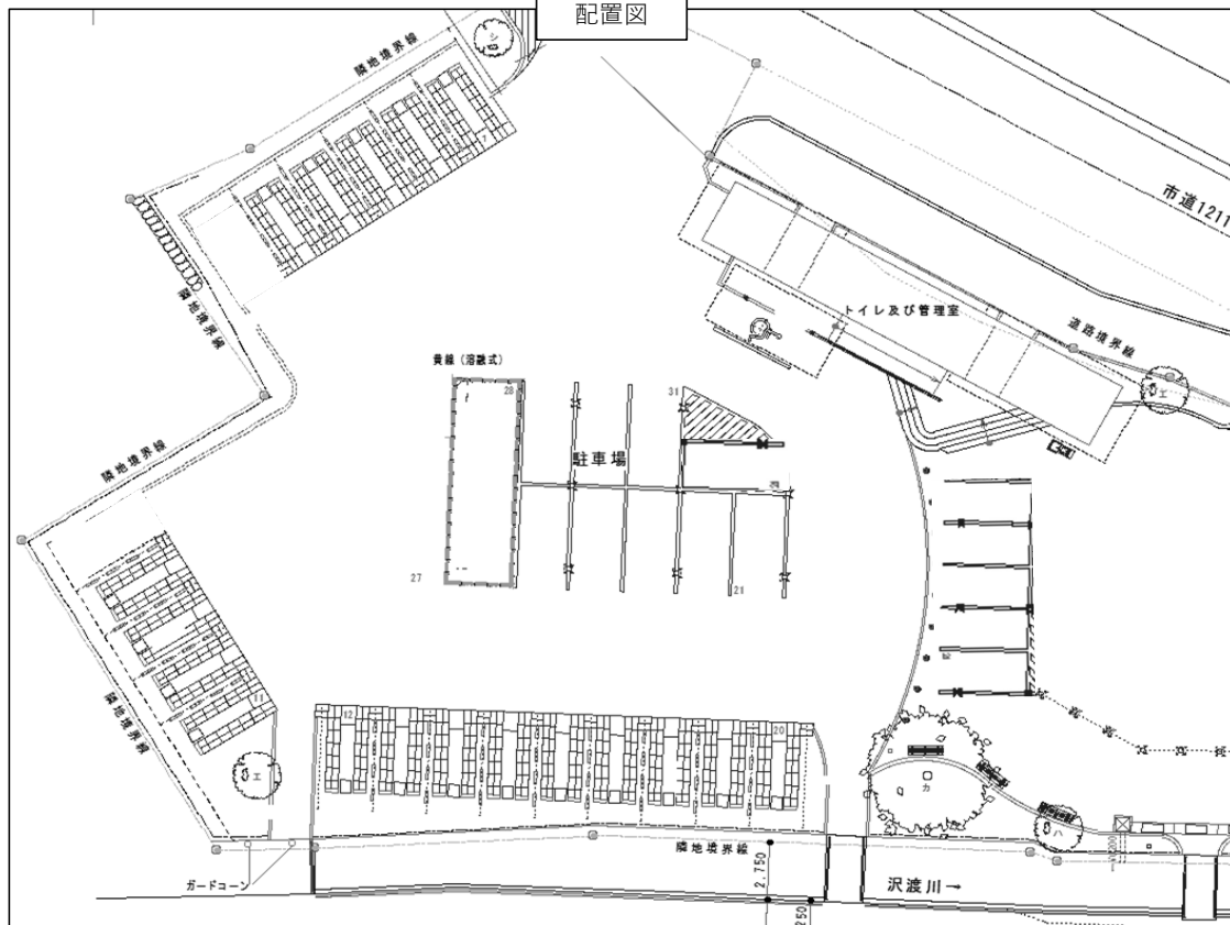
配置図
