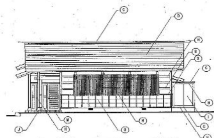
西側立面図 s=1/100
