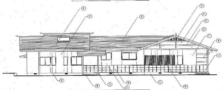
北側立面図 s=1/100
