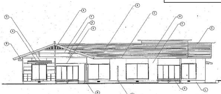
南側立面図 s=1/100
