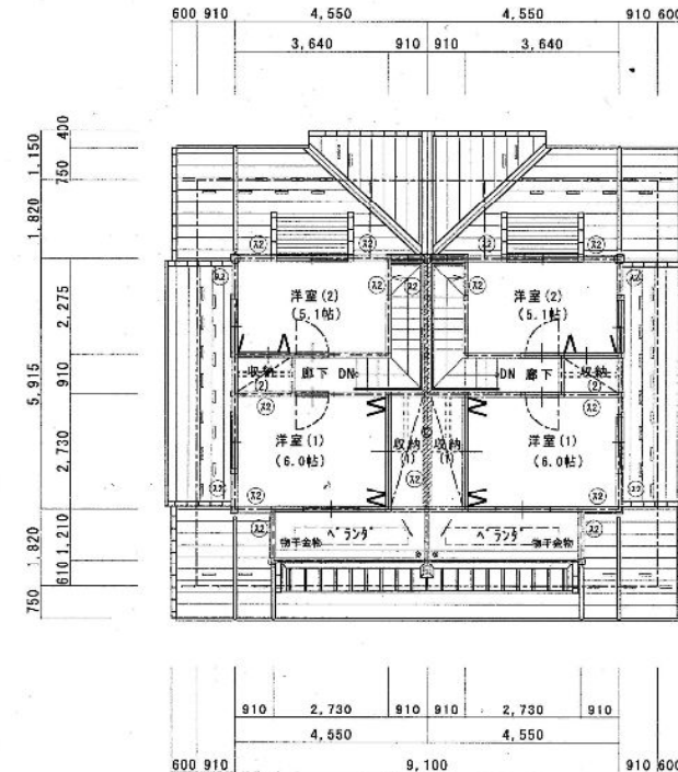
2階平面図
